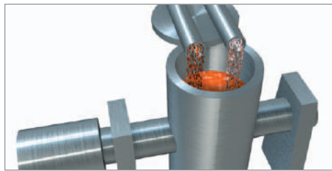
Processo di produzione delle guarnizioni in PTFE tradizionali
